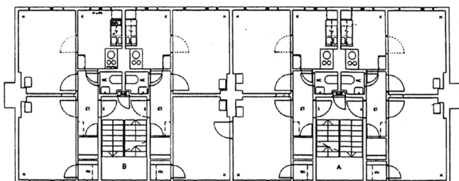
asuinkerroksen pohjapiirros 1:250
